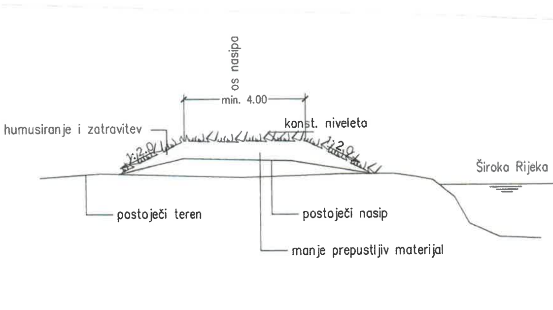
Slika 2: presjek nasipa
