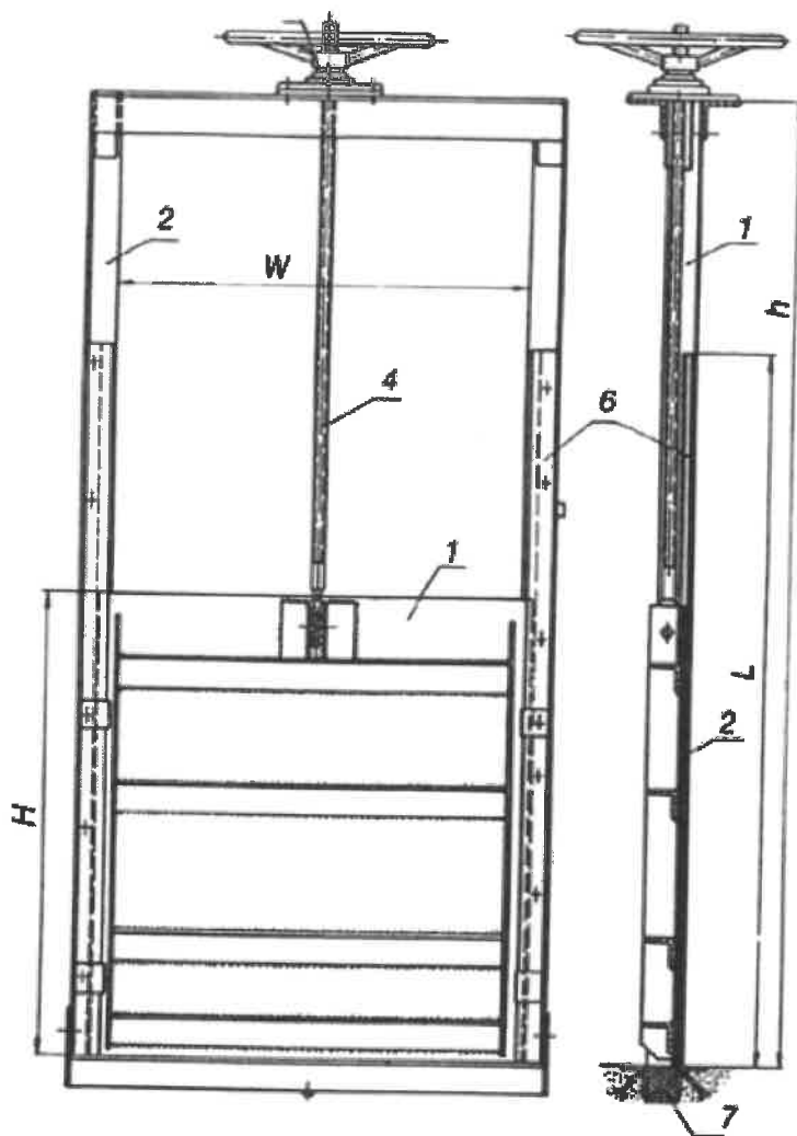
Slika 3: Zapornički mehanizam
