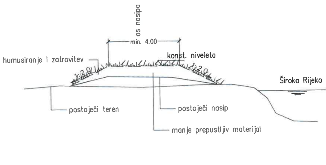
Slika 2: presjek nasipa
