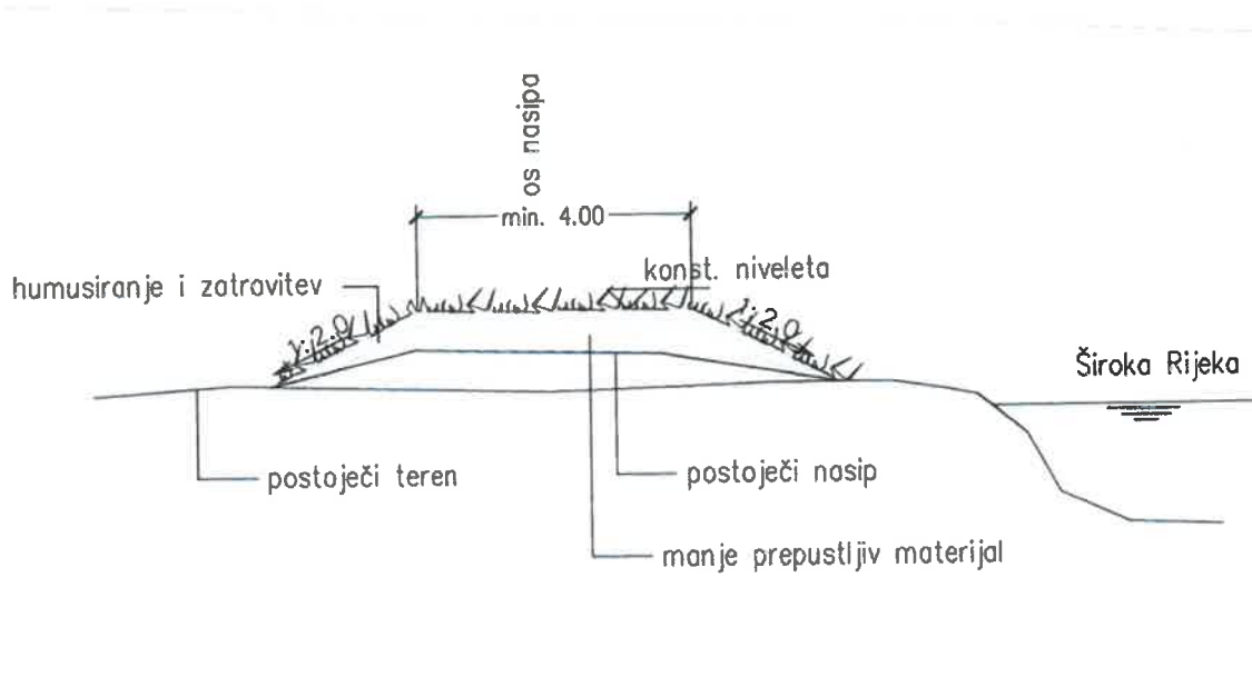
Slika 2: presjek nasipa
