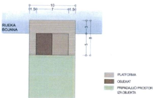
Slika: Princip postavljanja vikend kućice na vodi u odnosu na liniju obale i lokaciju
