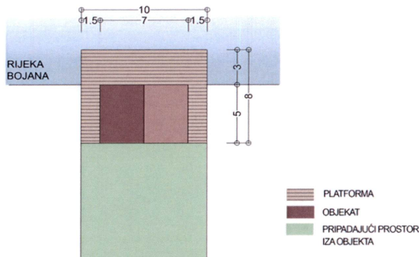
Slika: Princip postavljanja vikend kućice na vodi u odnosu na liniju obale i lokaciju
